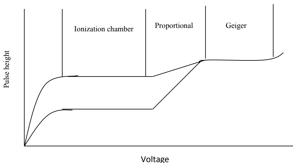
รูปที่ 2.14 กราฟของความสูงสัญญาณกับค่าโวลต์เทจคร่อมระหว่างหัววัดรังสีแบบแก๊ส แสดงถึงบริเวณอีออนไนเซชัน แคมเบอร์ บริเวณสัดส่วน และบริเวณไกเกอร์ ที่มา (โสรัชต์ เจริญวงศ์, 2530)
