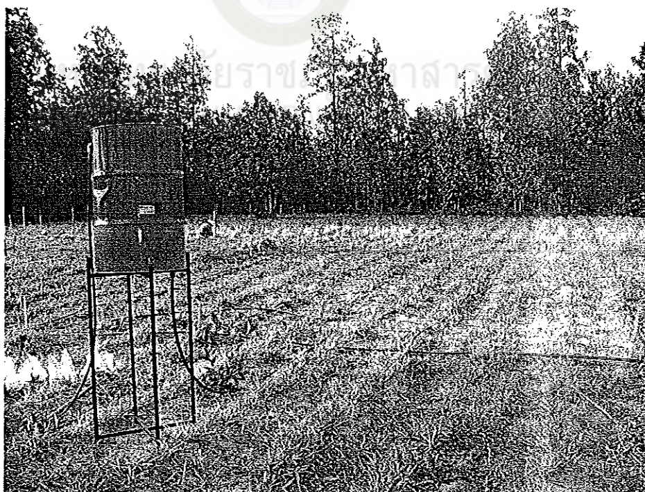
ภาพผนวกที่ 10 การวางระบบการให้น้ำแบบหยดในแปลงหญ้ารัฐ
